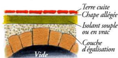
Solution maçonnée
